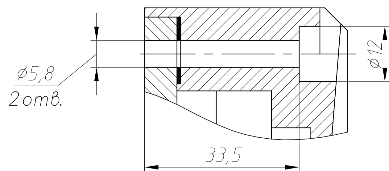
Б-Б(1:1)
