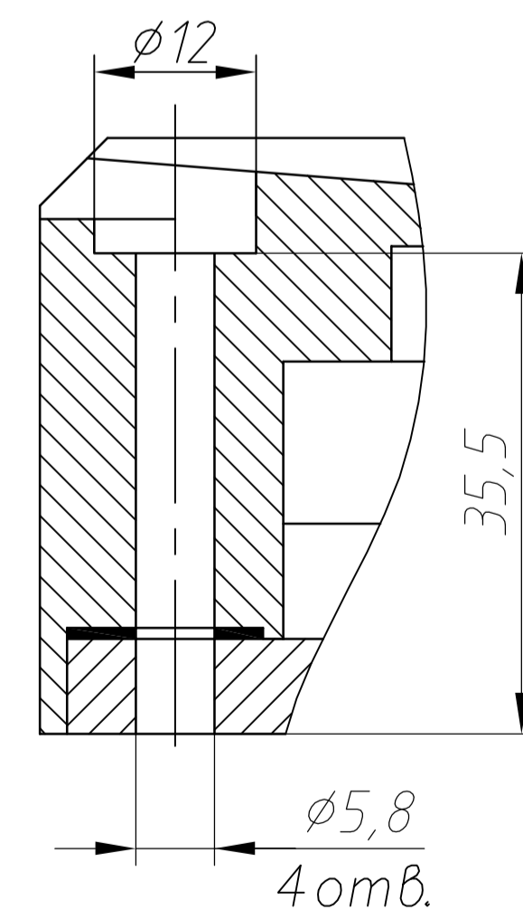
В-В(1:1)
